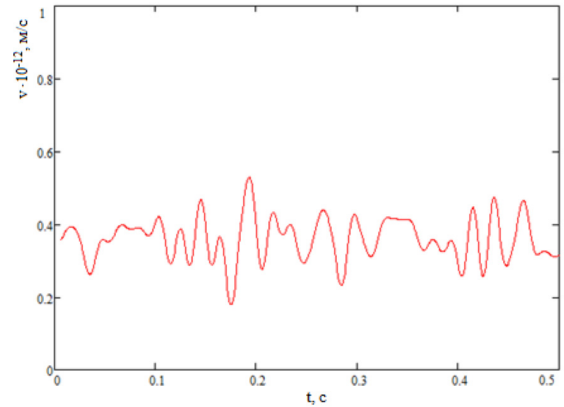
Рисунок 1.1 – Зависимость скорости движения наночастицы в поле лазерного излучения от времени ( n = 1,33 , \alpha = 0,53 , m = 5,5 \cdot 10^{-18} кг I_0 = 5,093 \cdot 10^6 Вт/м 2 , \lambda = 532 нм, v_0 = 10^{-3} м/с)
